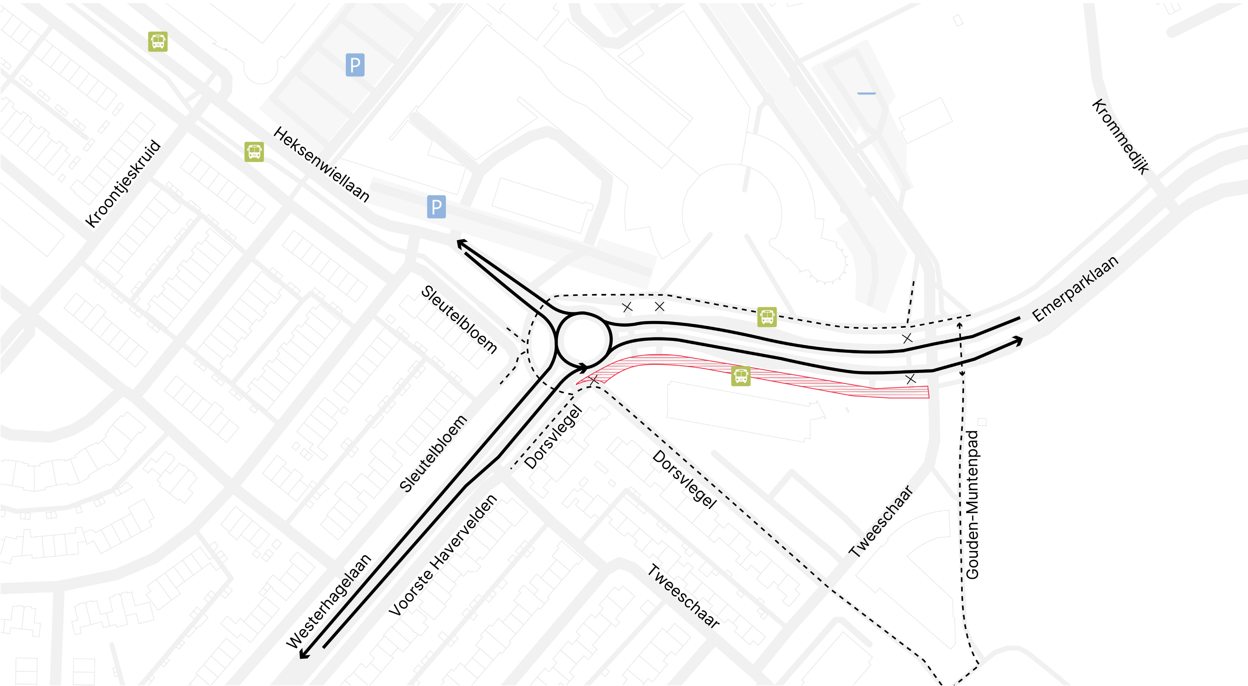
Fase 5 - Emerparklaan, fietspad zuid
